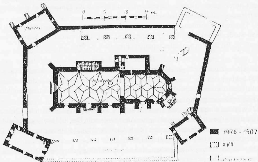
Grund- und Seitenrisse der Henndorfer Kirchenburg
